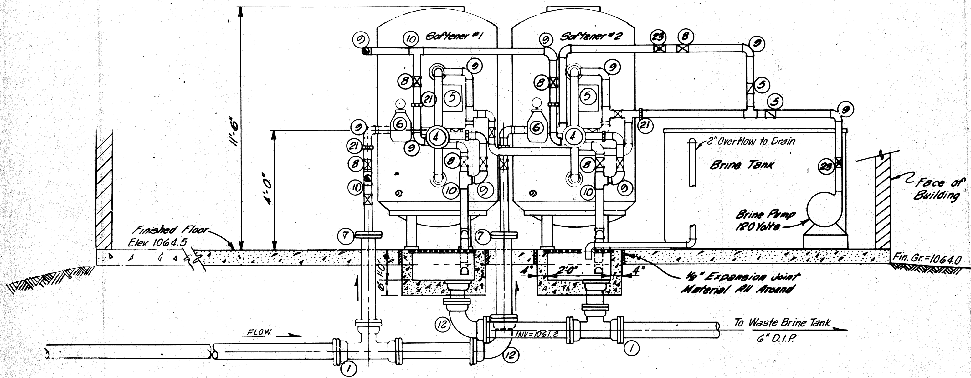
SECTION C-C Scale: 1/8" = 1'-0"
