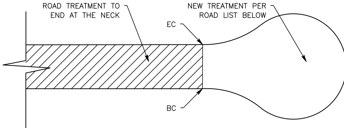
DETAIL 1 N.T.S
