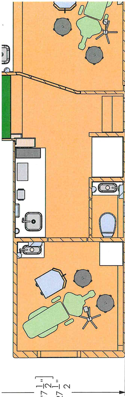
SECTION A-A SCALE 1 : 50
