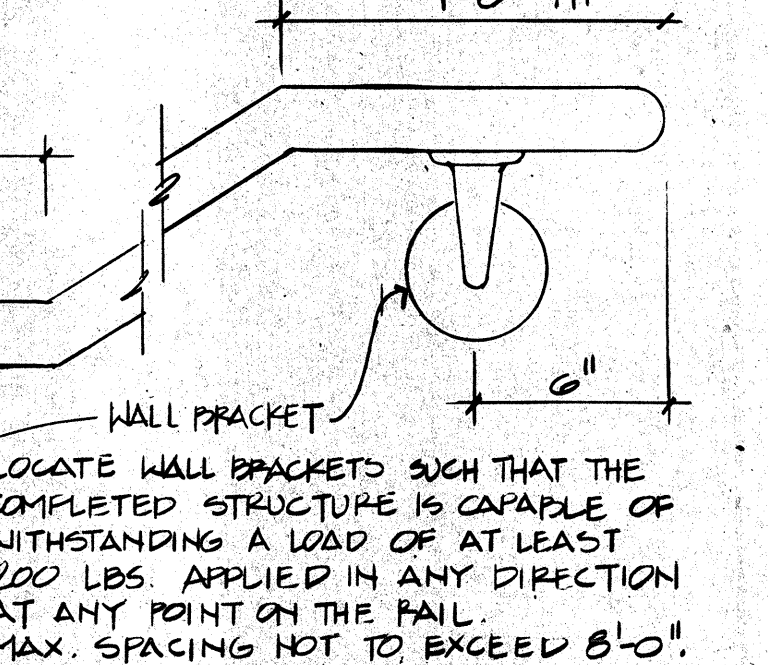
3 POST ANCHOR DETAIL SCALE: 3"=1'-0"
