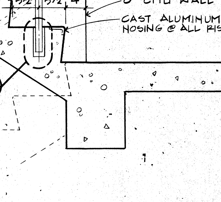
6 GUARDRAIL DETAIL SCALE: 1"=1'-0"
