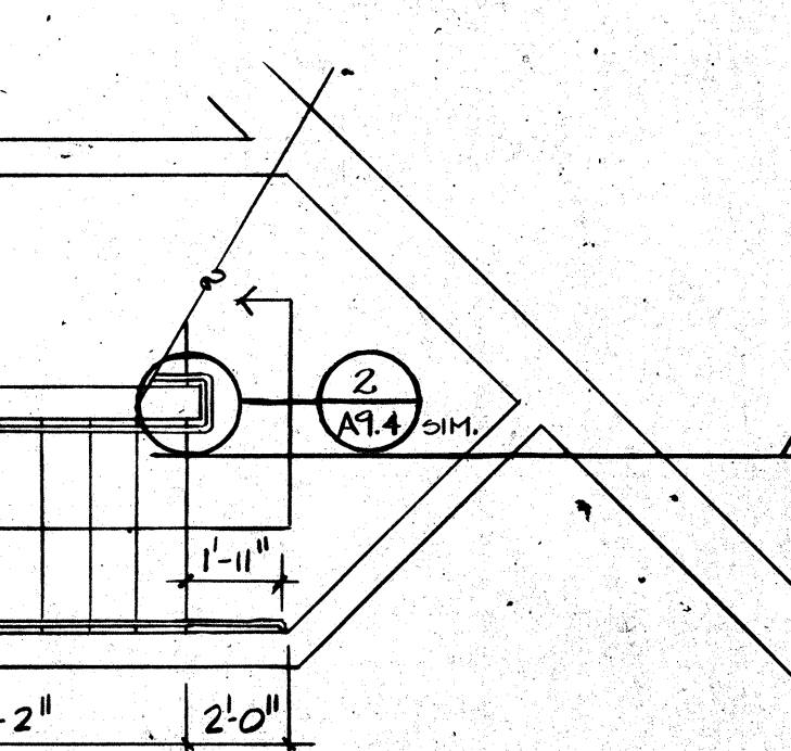
11 SECTION SCALE: 1/4"=1'-0"
