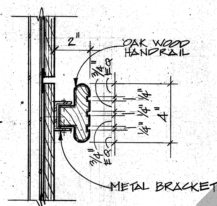
9 DETAIL SCALE: 3" = 1'-0"
