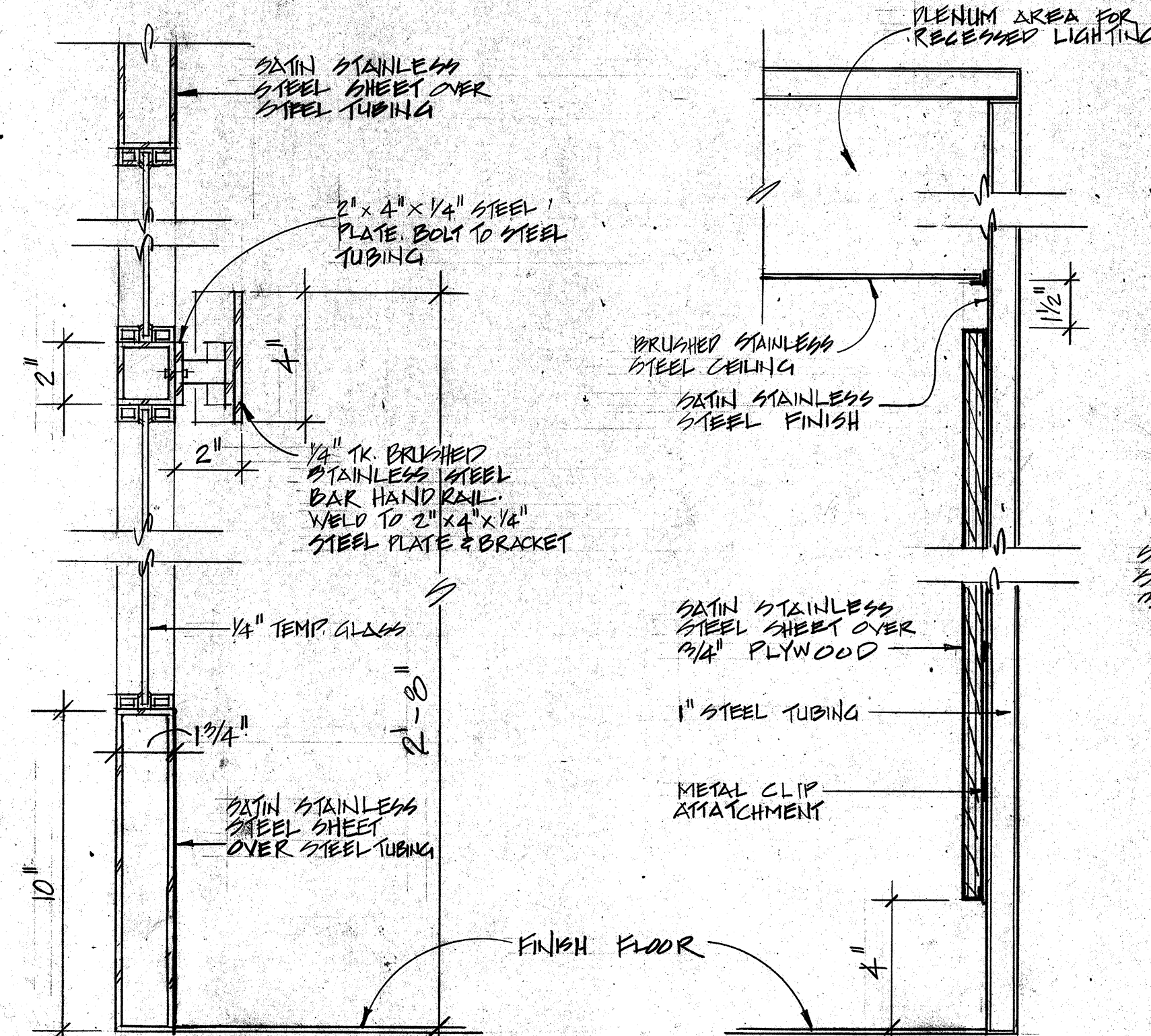
4 SECTION SCALE: 3" = 1'-0"
