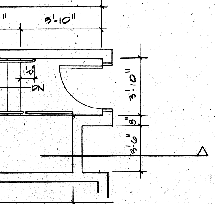
10 SECTION SCALE: 1/4"=1'-0"
