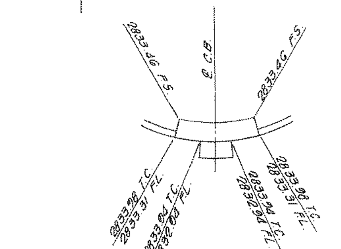
LOCAL DEPRESSION DETAIL SCALE: 1" = 20'
