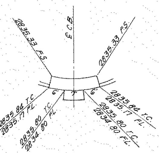
LOCAL DEPRESSION DETAIL SCALE: 1" = 20'
