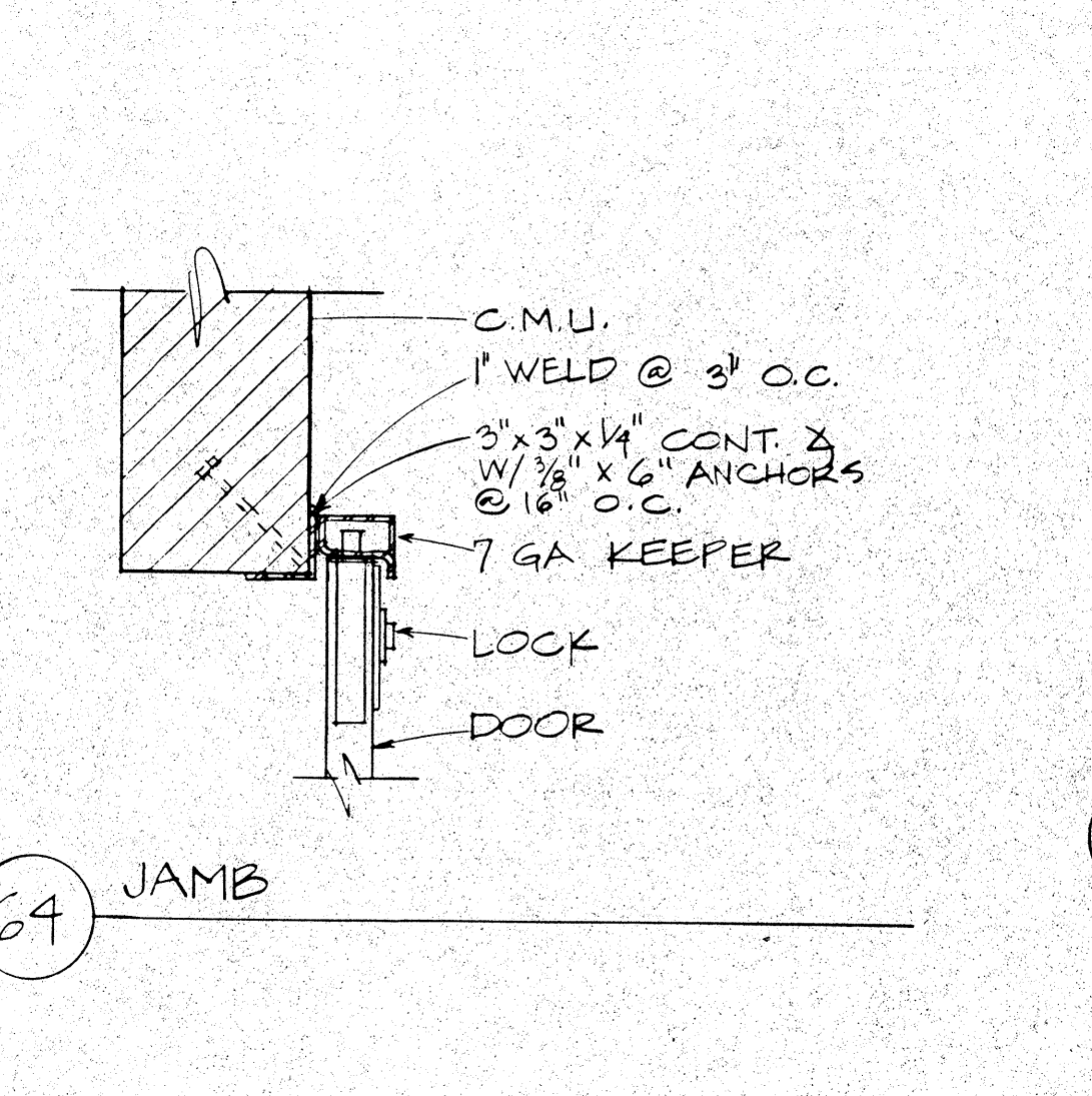
64 JAMB
