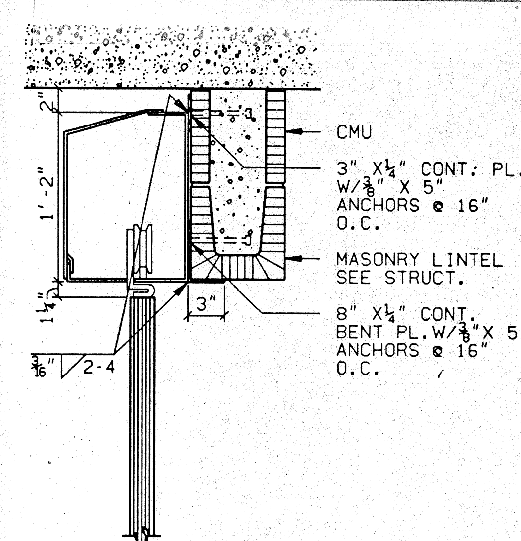
55 HEAD SCALE: 1 1/2" = 1'-0"
