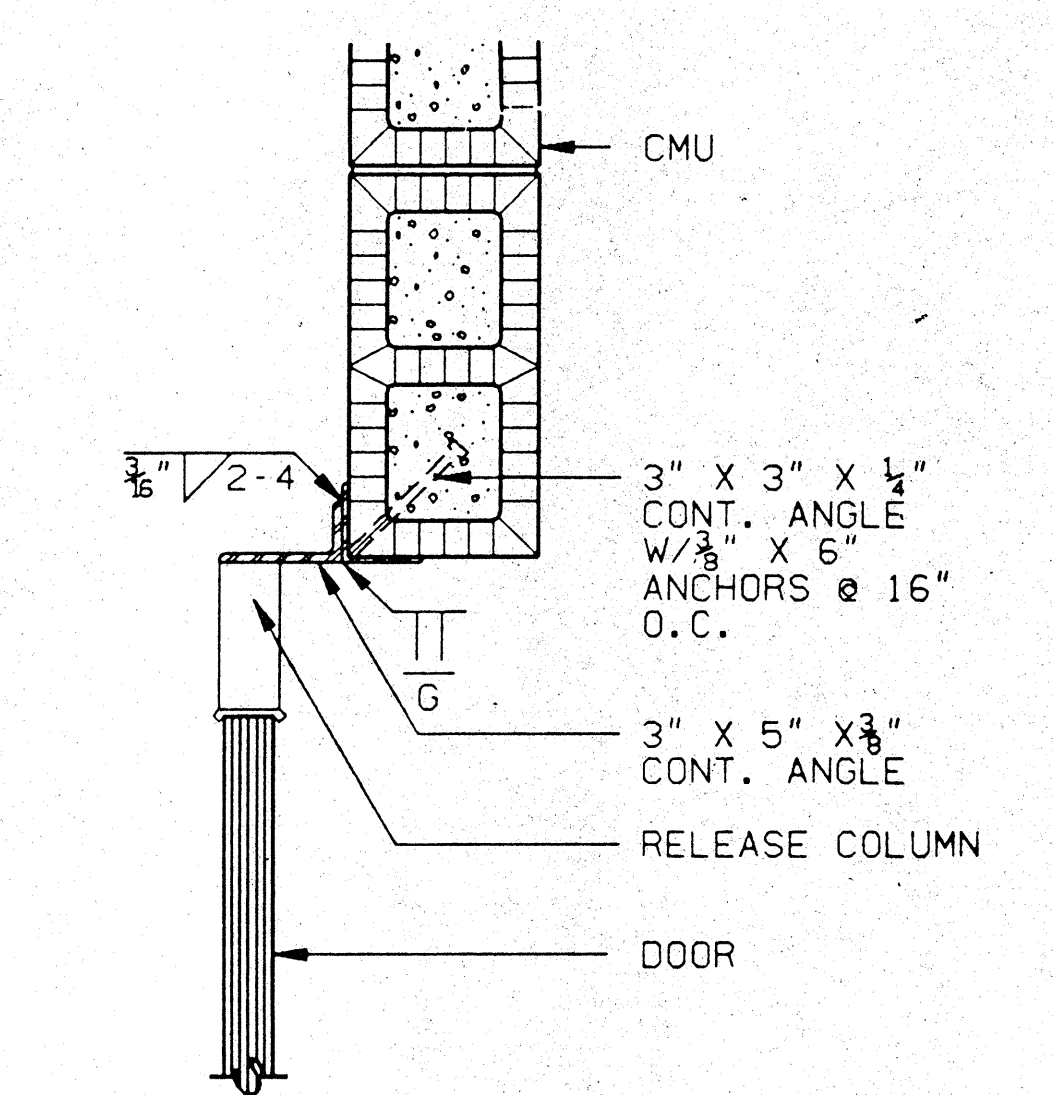
56 JAMB SCALE: 1 1/2" = 1'-0"
