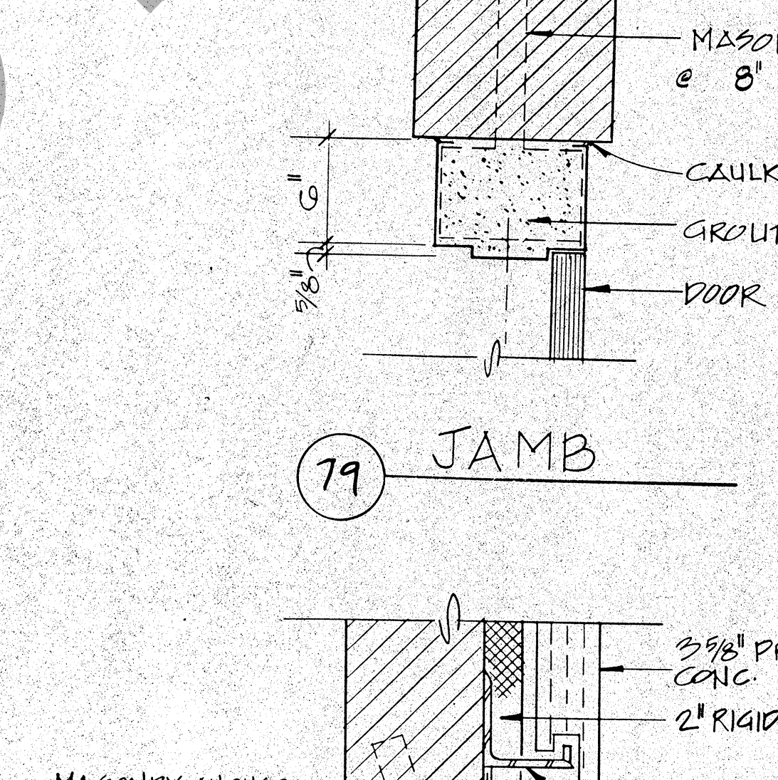
79 JAMB
