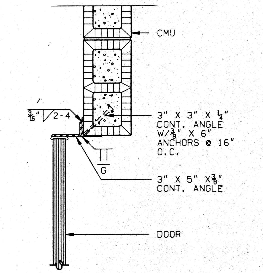
57 JAMB SCALE: 1 1/2" = 1'-0"
