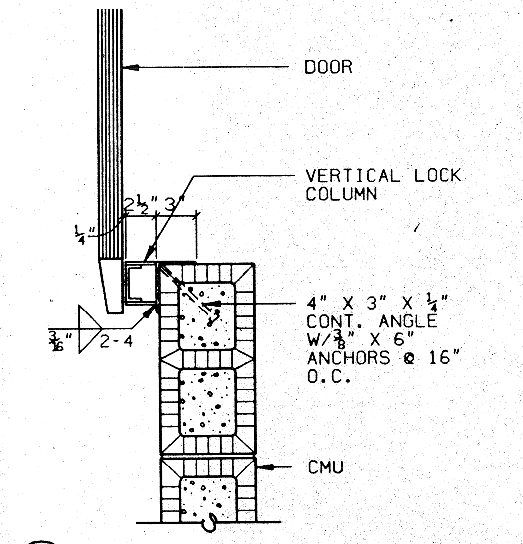
58 JAMB SCALE: 1 1/2" = 1'-0"
