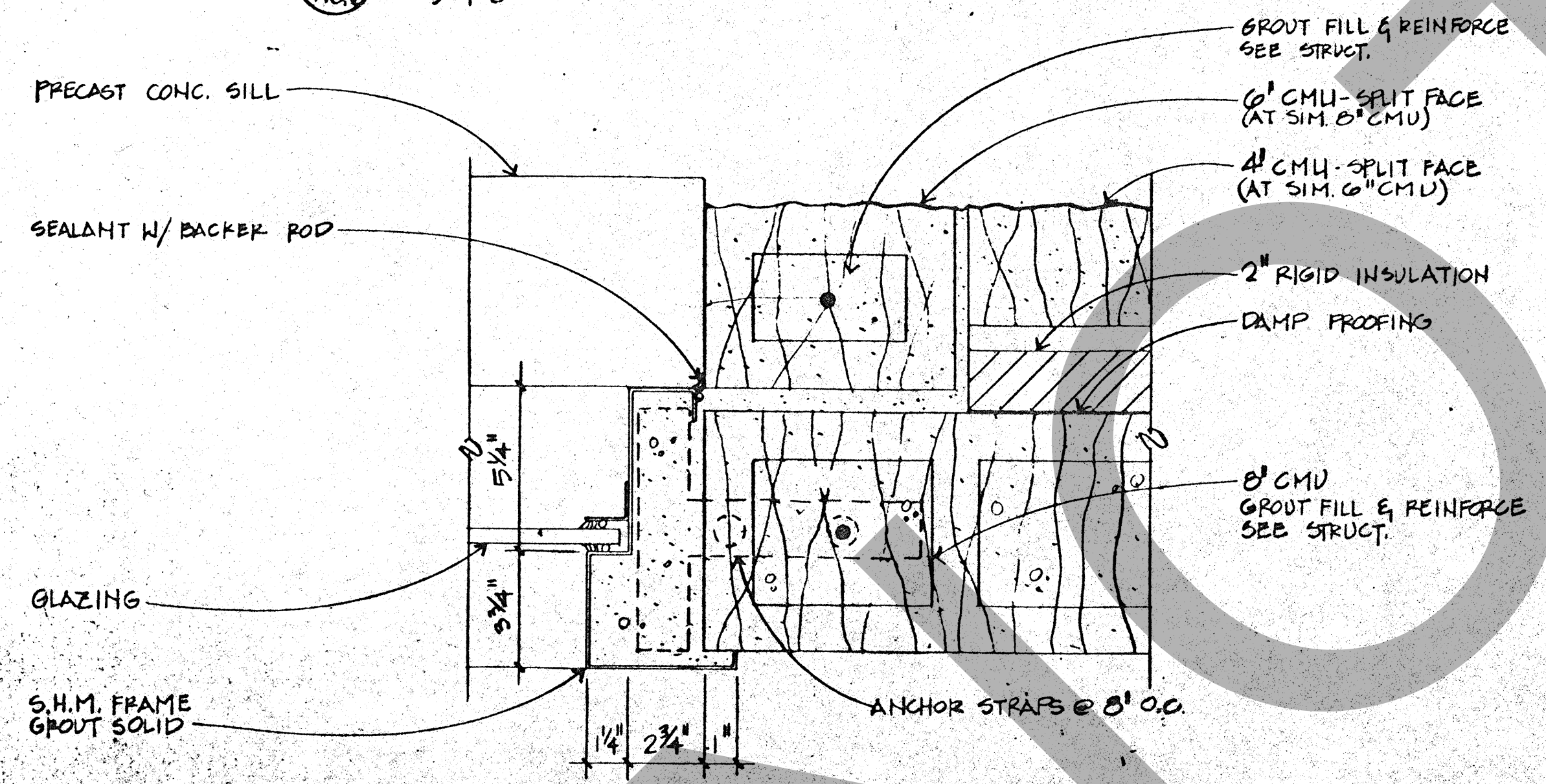
2 JAMB @ TYP. SECURITY WINDOW 3\"/>
