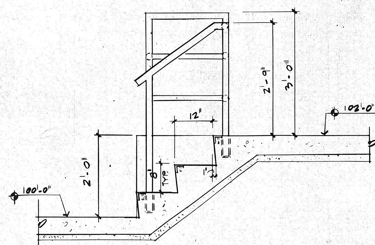
4 SECTION THRU STAIR SCALE: 1/4" = 1'-0"
